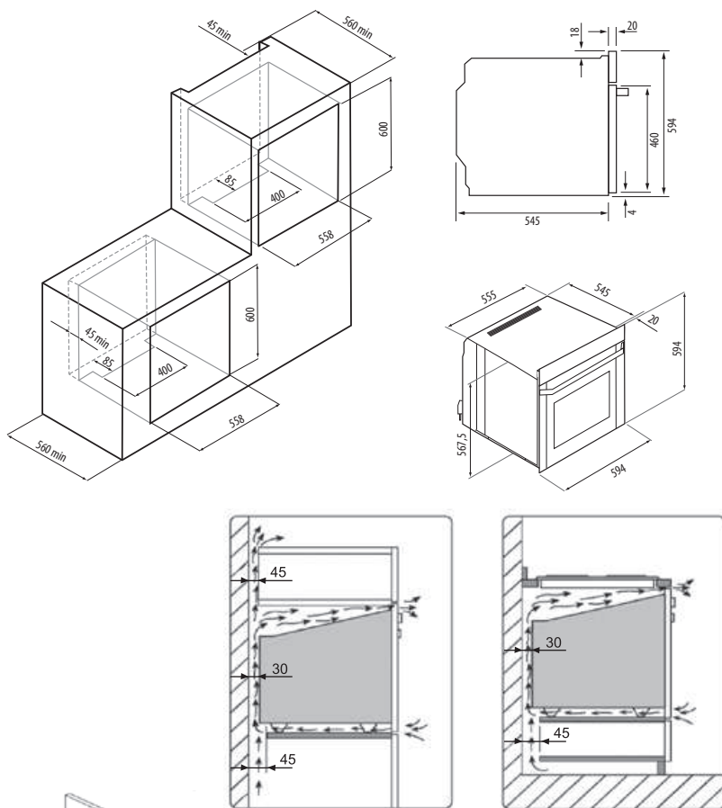
Рис. 6. Схема по встраиванию духового шкафа
