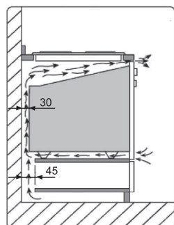
Рис. 6. Схема по встраиванию духового шкафа
