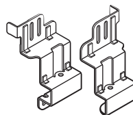
Набор кронштейнов для вертикальной установки (деталь № SK-DH)
