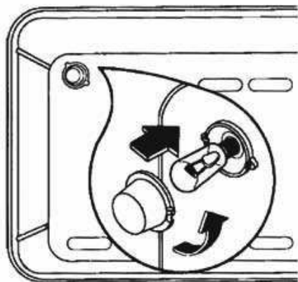
Рис. 8. Замена лампы
