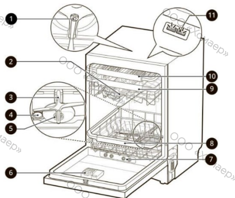
Вид изнутри
